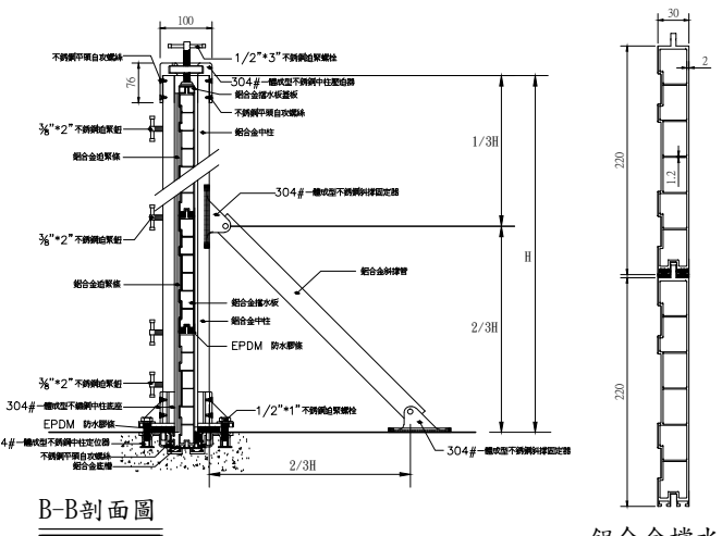
鋁合金擋水板
