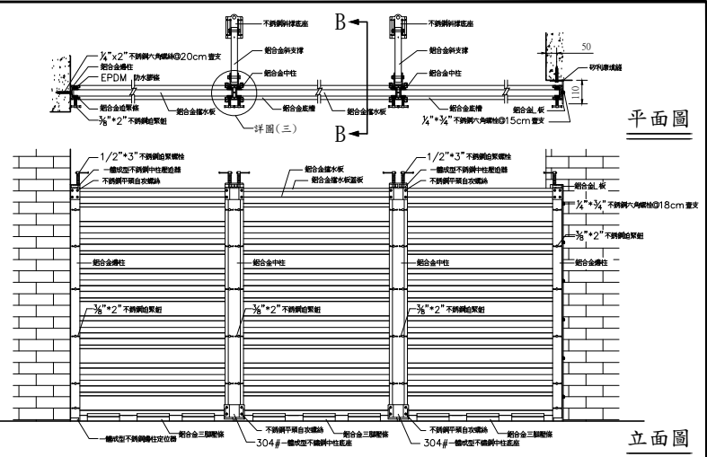
鋁合金擋水閘門(2支中柱)1內1外牆
