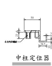
鋁合金擋水閘門(2支中柱)1內1外牆
