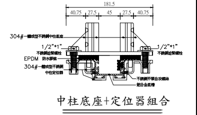
鋁合金擋水閘門(2支中柱)1內1外牆
