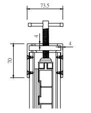
邊柱+壓迫器組合
