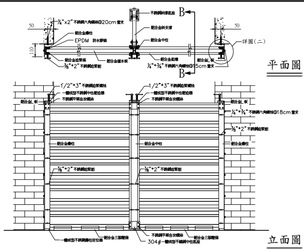
鋁合金擋水閘門(1支中柱)雙外牆
