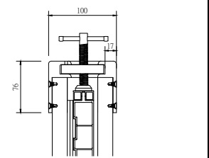
中柱+壓迫器組合
