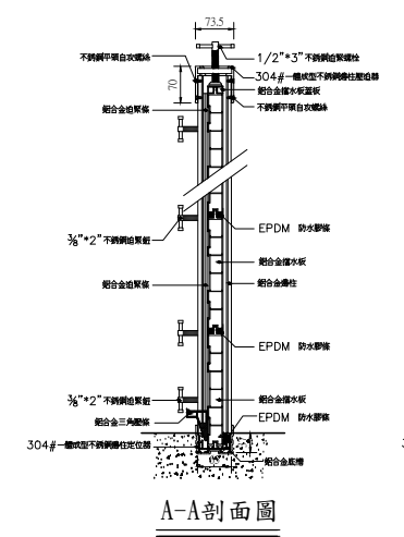
鋁合金擋水閘門(無中柱)雙內牆
