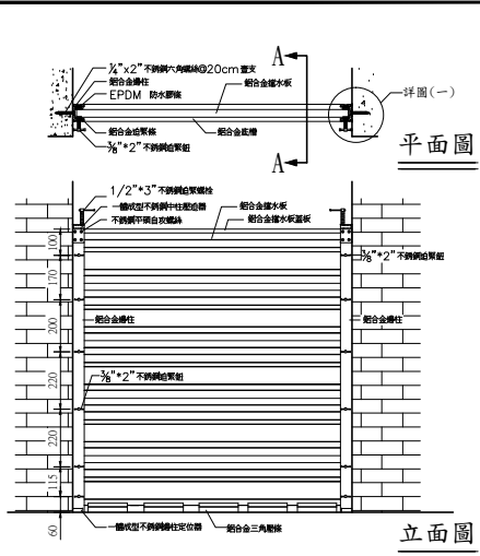
鋁合金擋水閘門(無中柱)雙內牆
