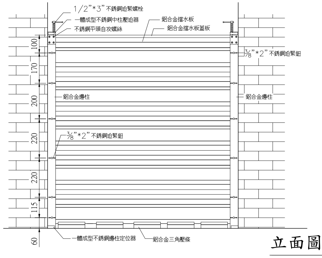
鋁合金擋水閘門(無中柱)雙內牆
